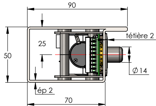
e-Profil : serrure 70172 & profil GT ou DP VUE DE DESSUS
